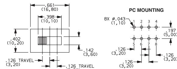
Actuator shown in pos. 1
